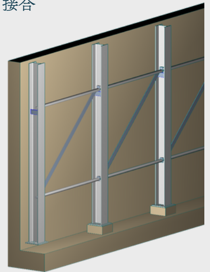
先行鋼製支保工に架ける
