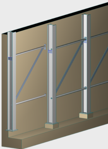
切羽内で先行鋼製支保工に誘導
